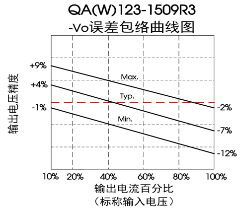
图 5 (辅路误差包络曲线)
