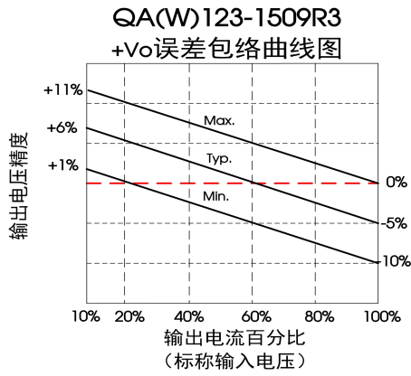
图 4 (主路误差包络曲线)
