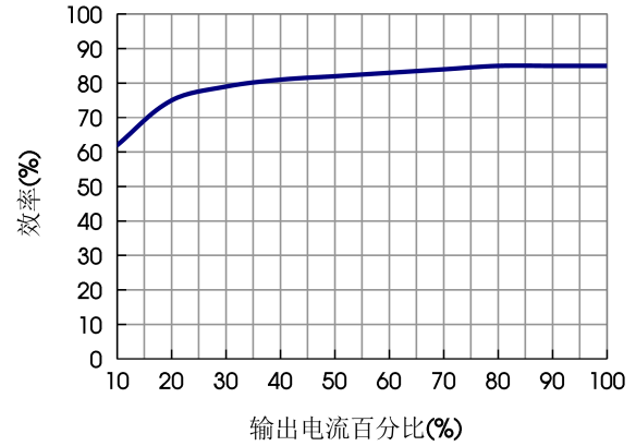
图 13(输出电流与效率关系曲线)
